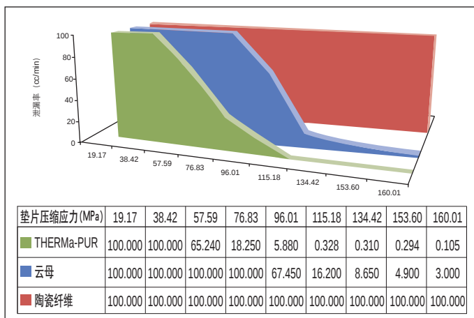
不同填充材料的缠绕垫片在不同压缩应力下密封性能对比
