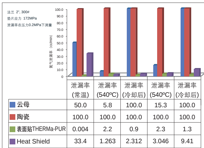
不同填充材料的缠绕垫片在热循环中的密封性能对比
